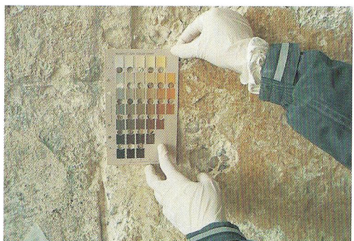
Estudio colorimétrico de paramentos exteriores e interiores basándose en pigmentos originales mediante colorímetro y cartas Munsell e Internacional.
